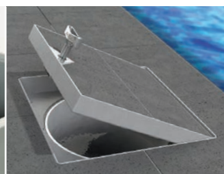
Action de rotation et de levage pour un accès facile aux boîtes d'écumoire
